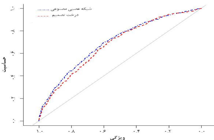
شکل ۴: سطح زیر منحنی راک برای مدل شبکه عصبی و درخت تصمیم در داده های آزمایشی
